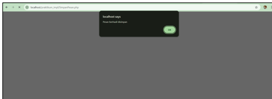
Gambar 1. 2 SimpanPesan.php
