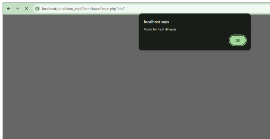
Gambar 2. 2 FormHapusPesan.php
